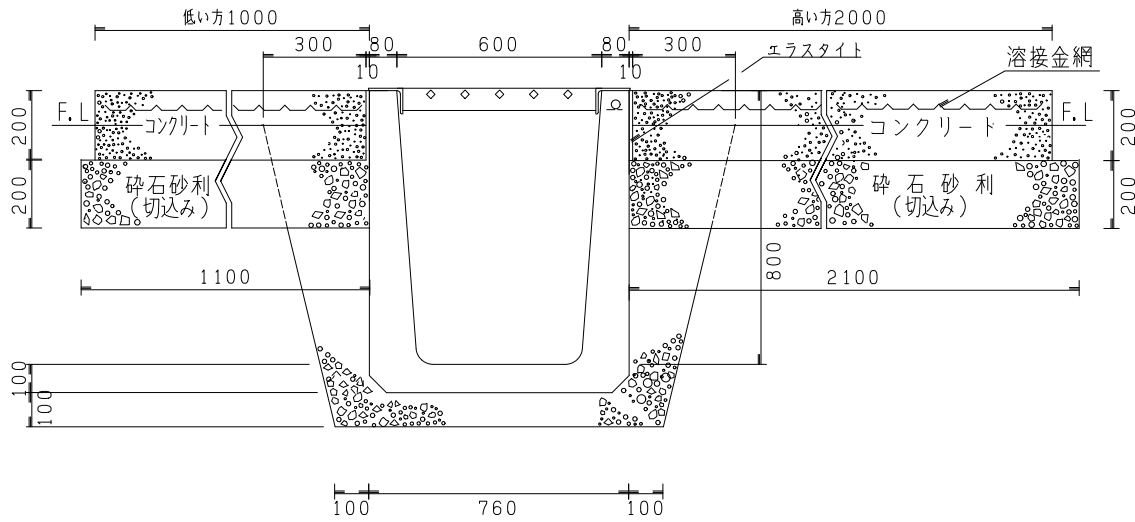
正面図 (断面) 土工定規図・構造図 (標準)
