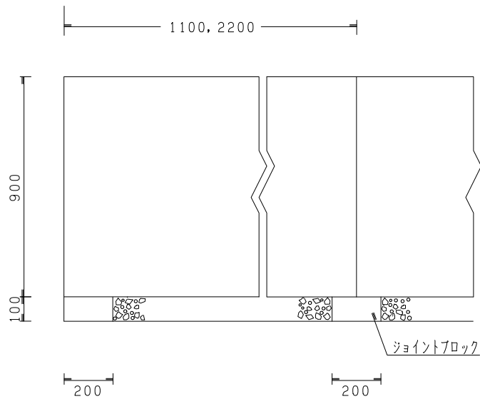
同上側面図
